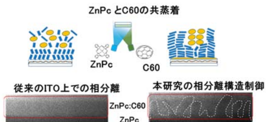
図 有機系太陽電池の写真(上左)、製膜に使う真空蒸着装置の写真(上右)、従来のITO上(下左)と本研究の無機半導体層上(下右)に共蒸着で製膜したバルクヘテロ層の断面電子顕微鏡写真。従来は均一に混合したものが、CuI上では柱状になっている。これは、無機半導体のd軌道と有機分子のπ軌道の相互作用で、有機分子スタックが横向きに変わり、スタックが変わることでバルクヘテロ構造の相分離が柱状の理想構造となった。
