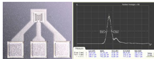
CMOS 技術による高速光検出器
