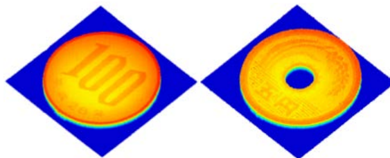
FMCW 光距離センサによる硬貨の 3D 計測
